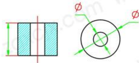
补偿套尺寸
