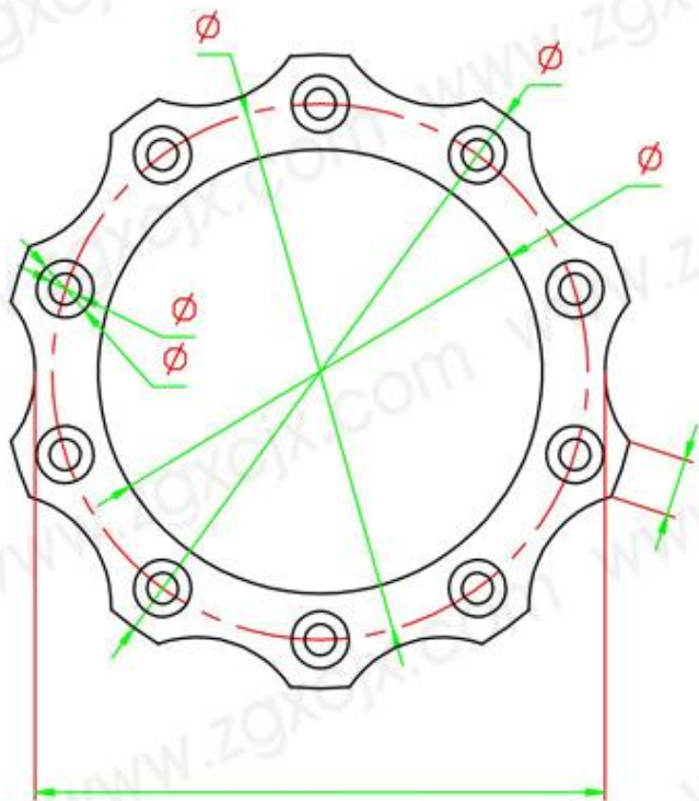
膜片尺寸
