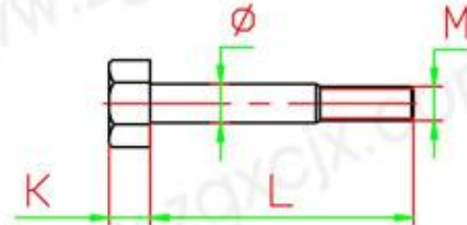
螺栓尺寸
