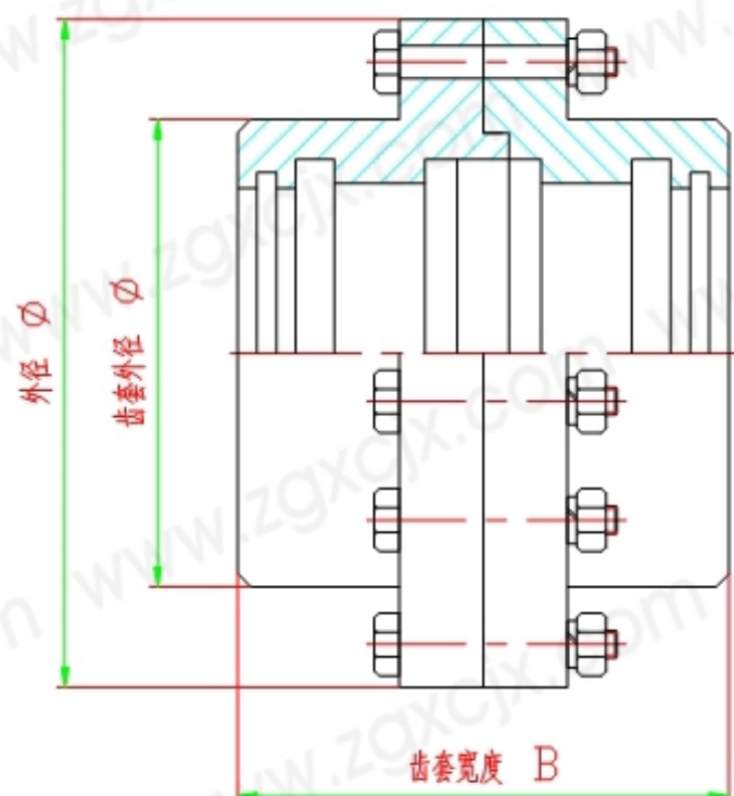
齿套
