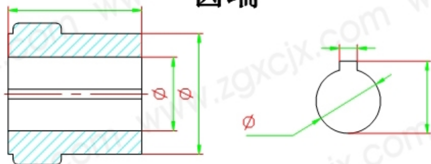
齿端
