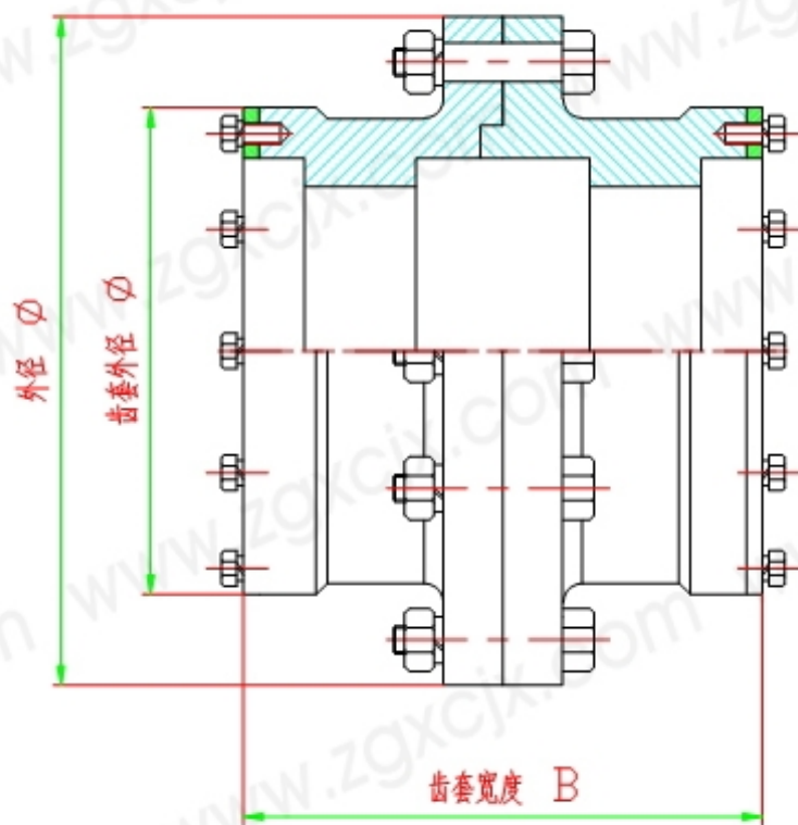
齿套
