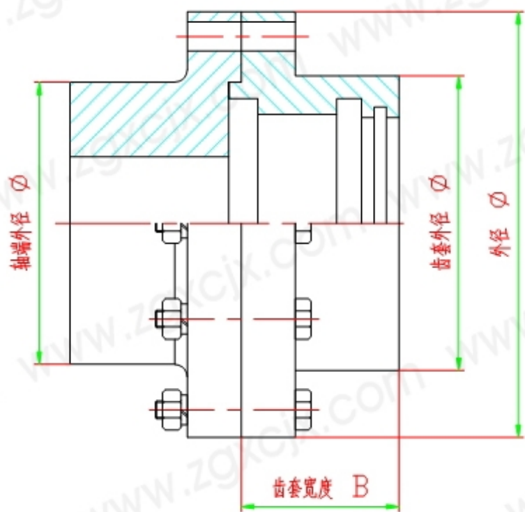
齿套
