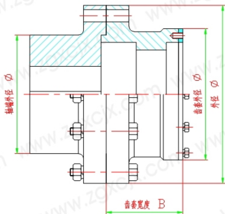
齿套
