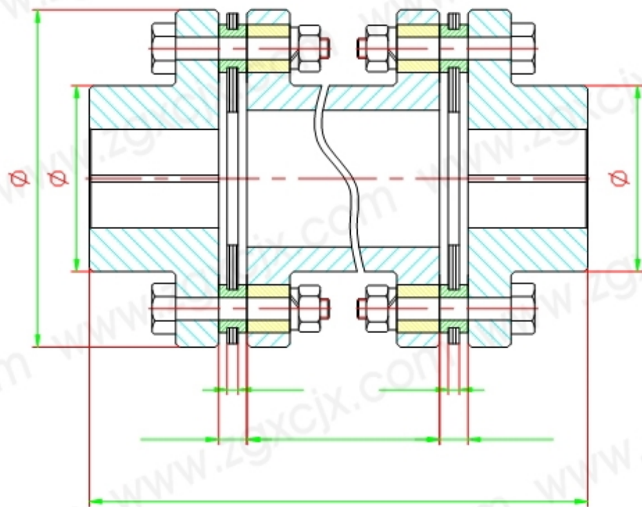
外形尺寸
