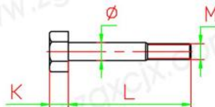
螺栓尺寸
