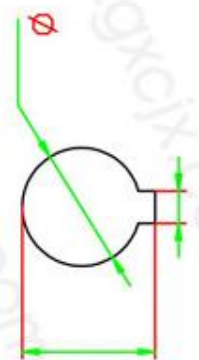
主动端
