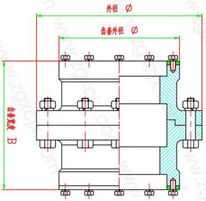
齿套
