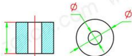
补偿套尺寸
