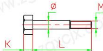
螺栓尺寸
