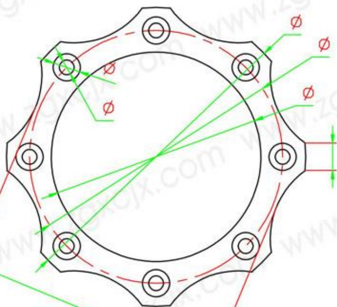
膜片尺寸
